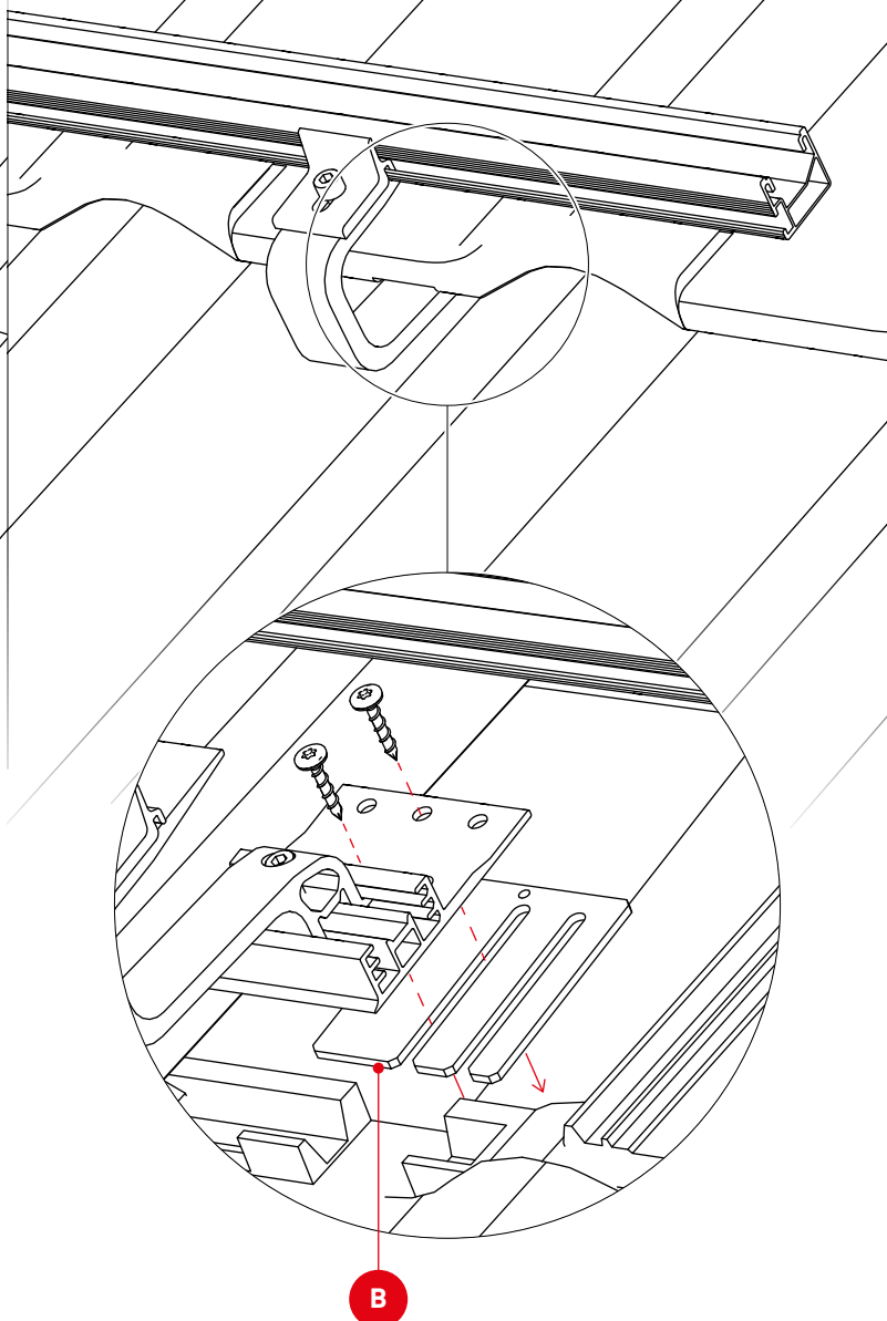
2002332 Cârlig de acoperiș placă de compensare 4 mm
